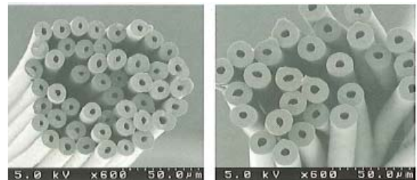
ダルチューブ®の糸断面
